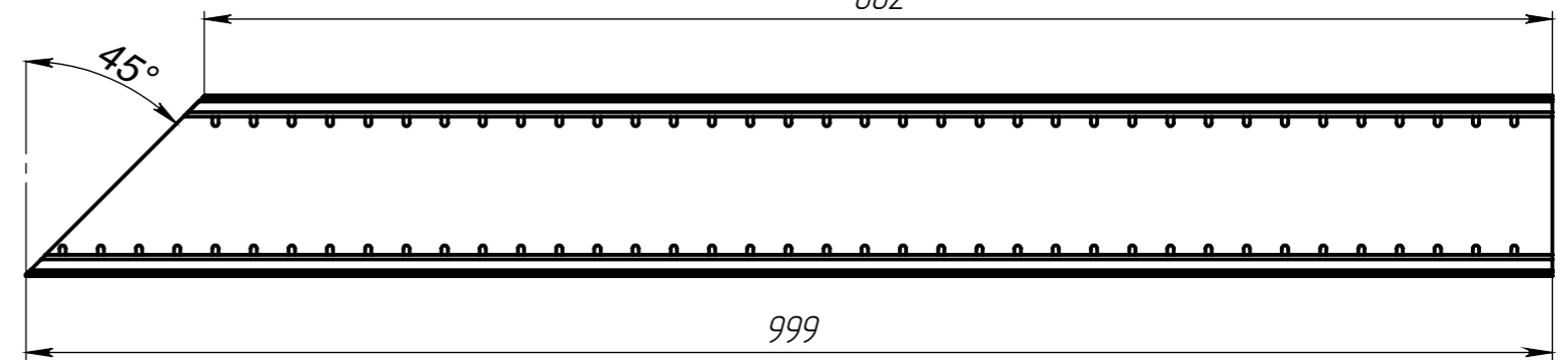
Вид сверху M(1:5)
